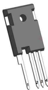
TO247-4
